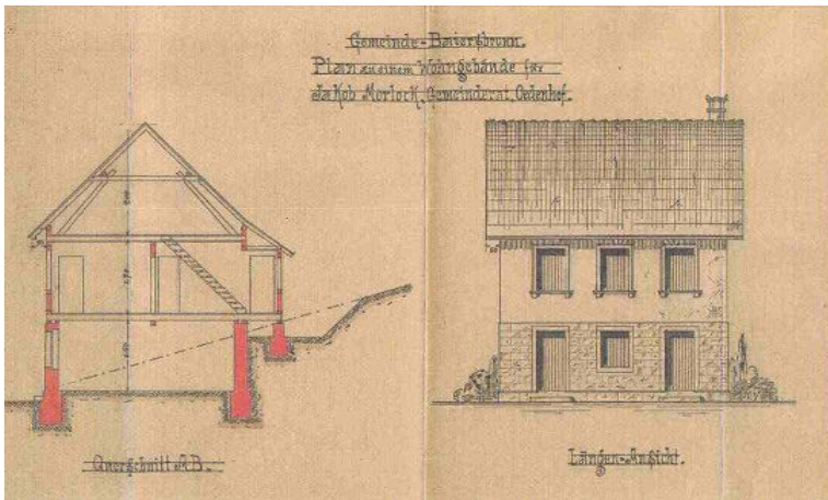
Plan des Austragshauses aus dem Jahr 1897
