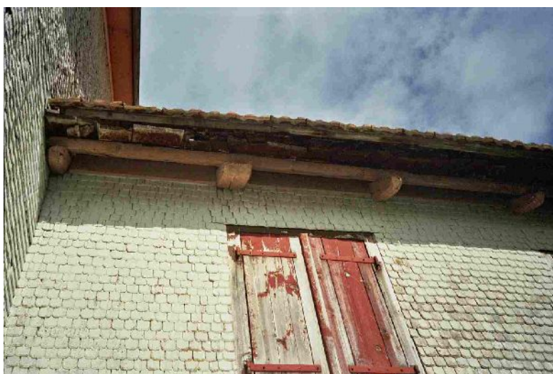
Ansicht der bauzeitlichen Traufe unter dem doppelt gedeckten Dach
