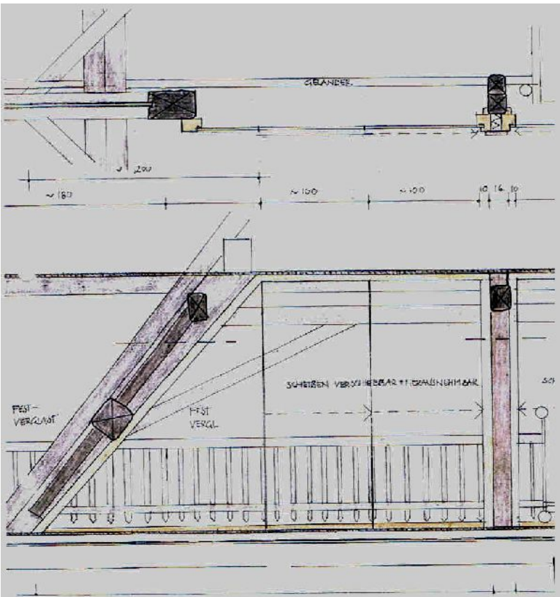
Detailzeichnung für die gläsernen Schiebetüren
